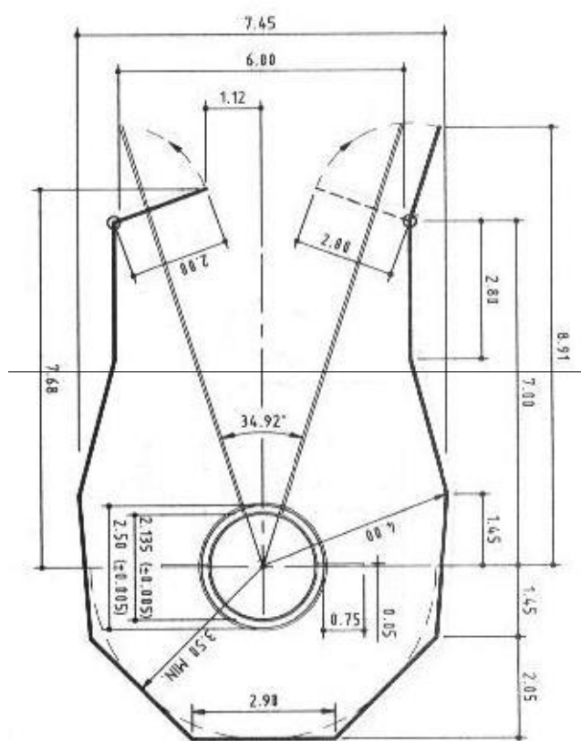
Obr. 192b - Klec se soustřednými kruhy pro hody diskem a kladivem nastavená pro hod kladivem
