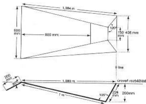
Obr. 183a - Skříňka pro skok o tyči
