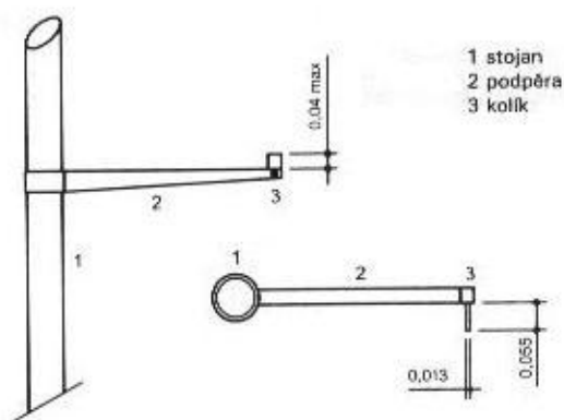
Obr. 183b - podpěry pro laťku
