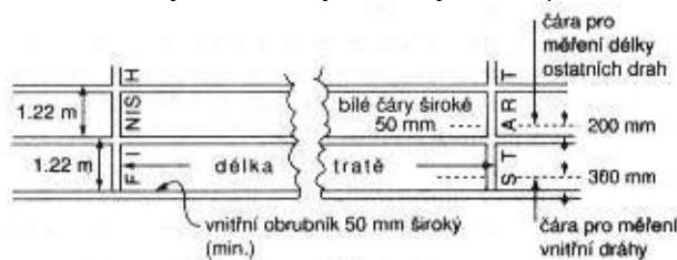
Obr. 160 – Měření délky dráhy
